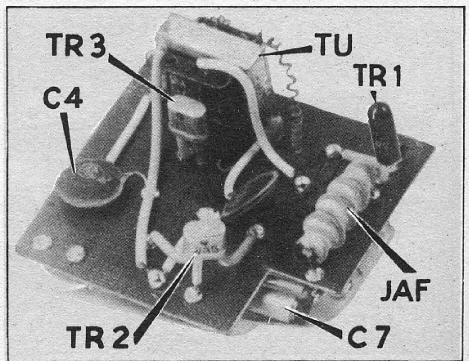
Due vedute del pannello chassis nell'altra versione
